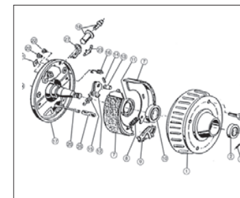
Hjulbroms RM 2051 / T 070 Ps
