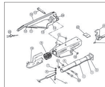
Påskjutbroms 100s / T 068 Ps
