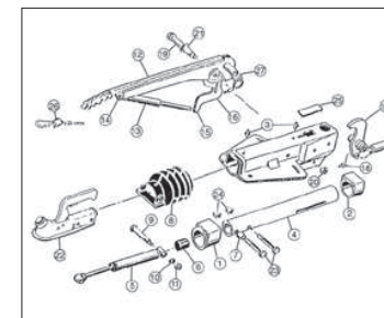
Påskjutbroms 161s / T 069 Ps
