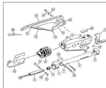
Påskjutbroms 251s / T 084 Ps
