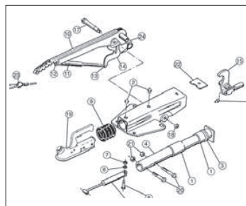
Påskjutbroms 100s / T 067 Ps
