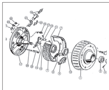
Hjulbroms RM 1637 / T 067 Ps
