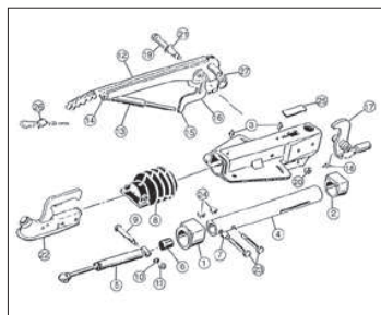
Påskjutbroms 161s / T 070 Ps
