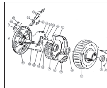
Hjulbroms RM 2051 / T 069 Ps
