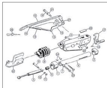
Påskjutbroms 161 / T 082 Ps
