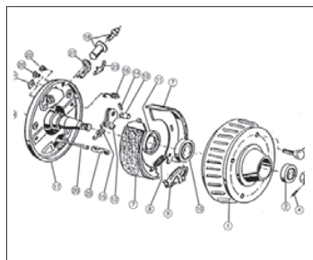
Hjulbroms RM 2361 / T 082 Ps
