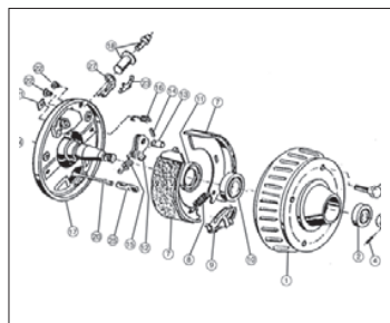
Hjulbroms RM 2051 / T 084 Ps
