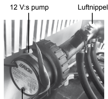
Vred för reglering av pumpens hastighet
