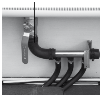
Shuntventil golvvärme i öppet läge
