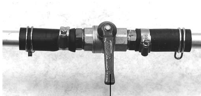
Shuntventil stängd
