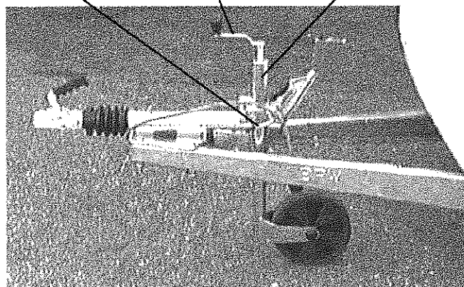
Låsvred för stödhjulsben Vev för höjning och sänkning av stödhjul Stödhjulsben
