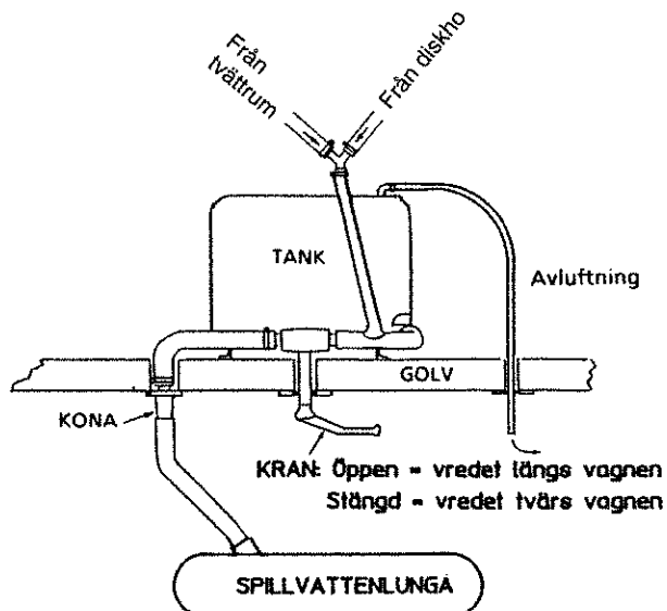
Avloppstank
