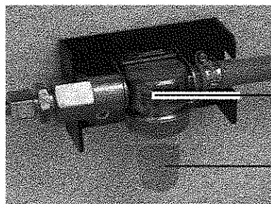
Läckindikator
