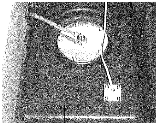
Avloppstank
