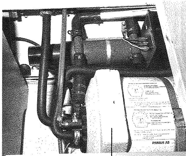
Varmvattenberedare
