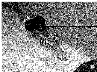
Avtappningskran varmvattenberedare (i stängt läge)
