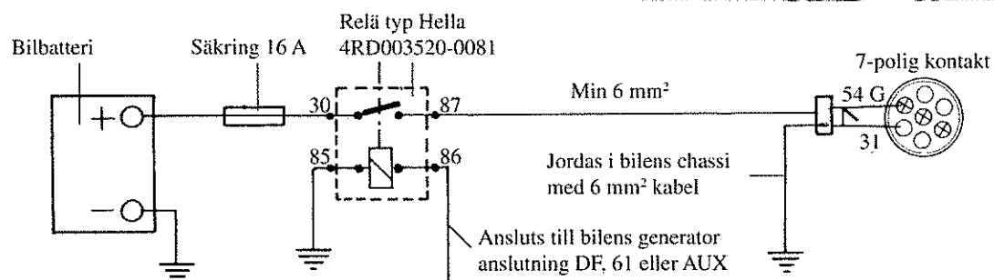
Schema som visar kopplingen i bilen vid laddning av vagnens batteri från bilens generator
