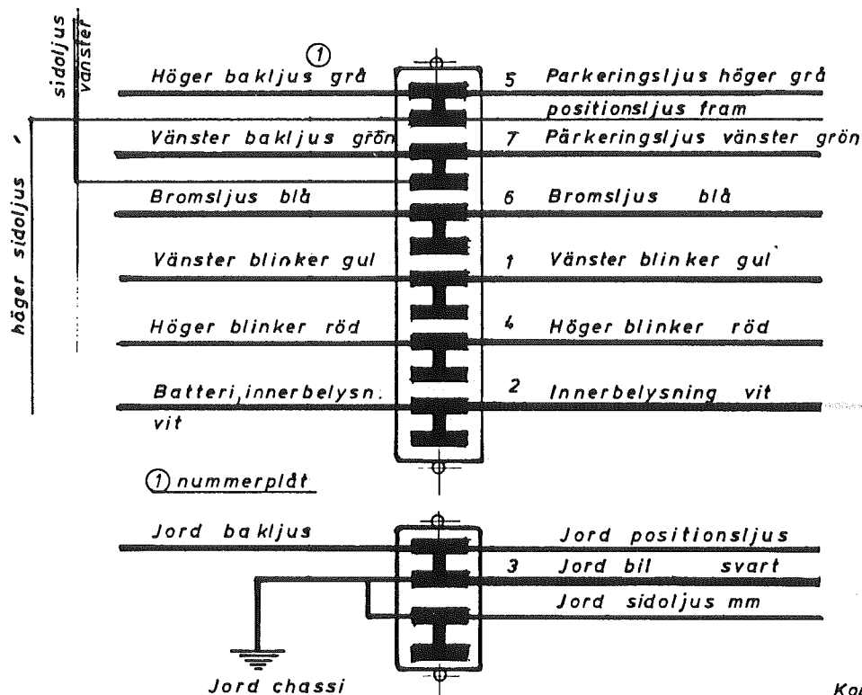
Husvagnens koppl. sedd från utsidan
