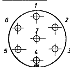
Bilens koppl. sedd från utsidan
