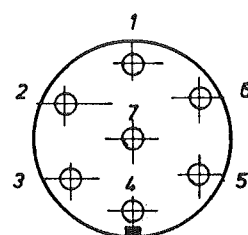
Husvagnens koppl. sedd från utsidan
