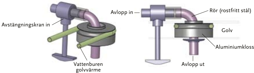
Den vattenburna golvvärmens värmer även avloppet, vilket säkerställer att det inte fryser på vintern.
